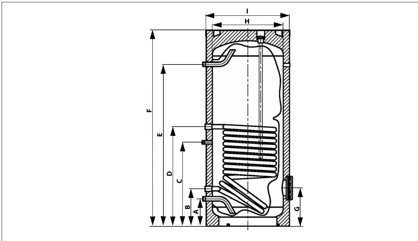
Snitbillede af HDG brugsvandsbeholder type RS
